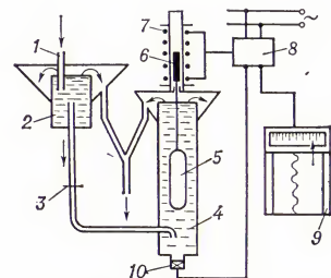
Рис. 1. Схема плотномера с плавающим поплавком: 1 — входная труба; 2 — переливной сосуд, обеспечивающий постоянство напора жидкости; 3 — диафрагма, устанавливающая скорость потока; 4 — измерительный сосуд с переливным устройством; 5 — металлический поплавок с сердечником; 6; 7 — индуктивный датчик, включённый в схему измерительного моста; 8; 9 — самопишущий прибор (или автоматический регулятор); 10 — термометр сопротивления для коррекции показаний на изменение температуры.
